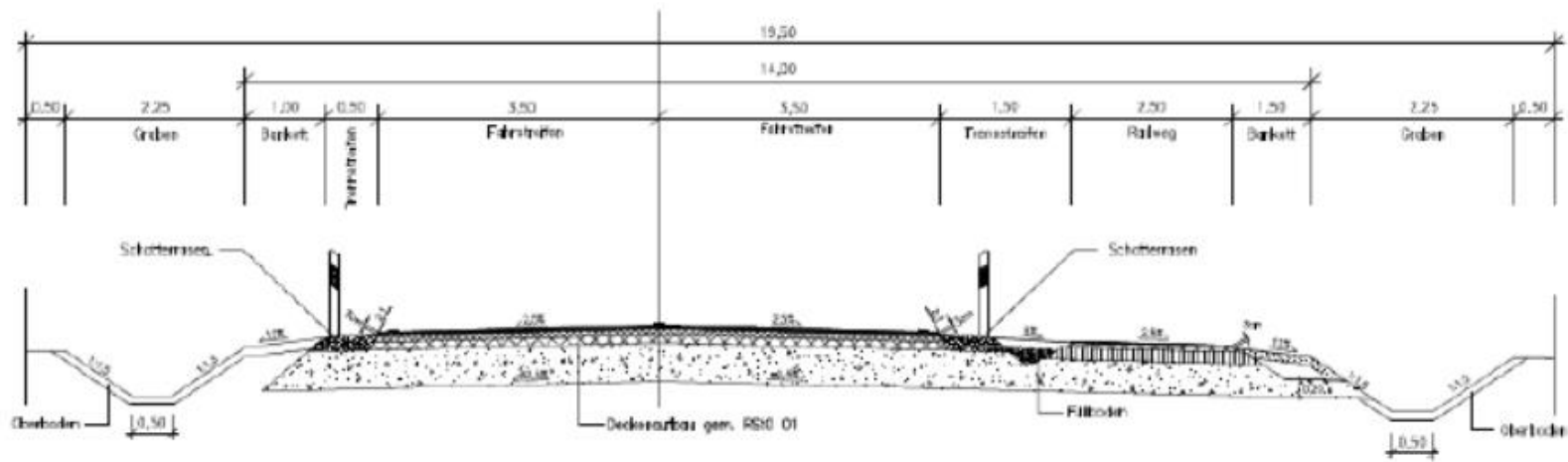
Abbildung 8 Regelquerschnitte [eigene Darstellung]
